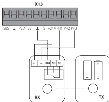
Рисунок 7. Підключення фотоелементів з батарейками, що спрацюють під час зачинення
