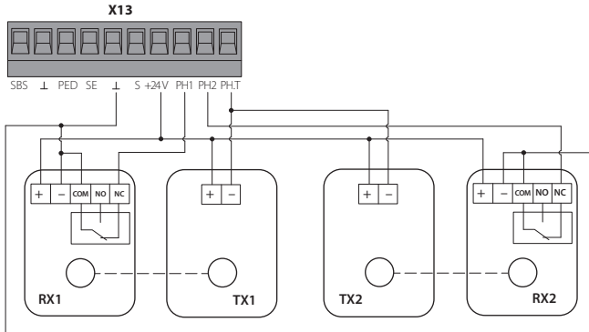
Рисунок 6. Підключення фотоелементів, що спрацюють під час зачинення та відчинення
