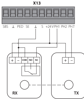
Рисунок 5. Підключення фотоелементів, що спрацюють під час зачинення
